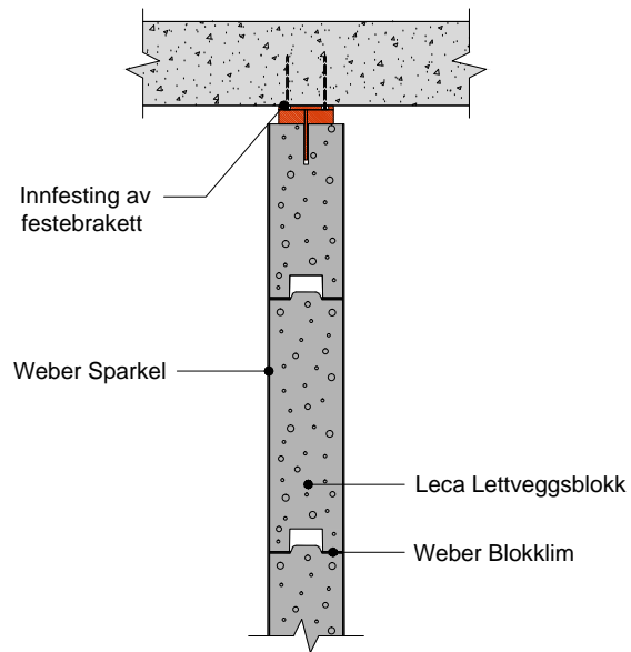
Snitt A-A - Innfesting mot etasjeskiller av betong med skjult festebrakett.
